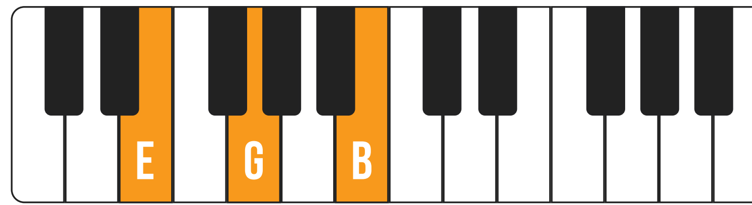
E minor (Em)
